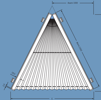
SDP 3: En, Yükseklik, Sol eğim, Sağ eğim
