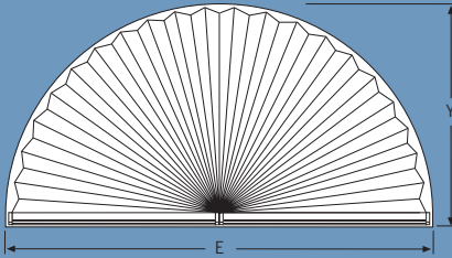
SDP 2: En, Yükseklik, Eğim
