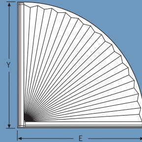
SDP 3: En, Yükseklik, Sol eğim, Sağ eğim
