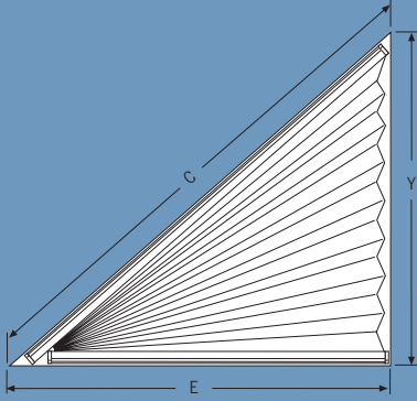
SD 2: En, Yükseklik, Eğim
